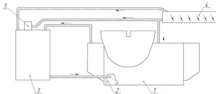
Рис. 3. Схема роботи системи охолодження охолоджуючої рідини дизеля типу 5ТДФ
