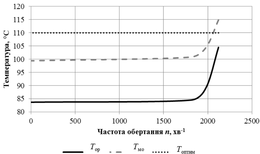
Рис. 5. Результати експерименту ДП «ХКБМ»: температури охолоджуючої рідини та оливи від частоти обертання і навантаження на дизель типу 5ТДФ
