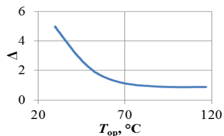
Рис. 1. Відносний знос циліндрів дизеля типу 2Д100 в залежності від температури охолоджуючої рідини
