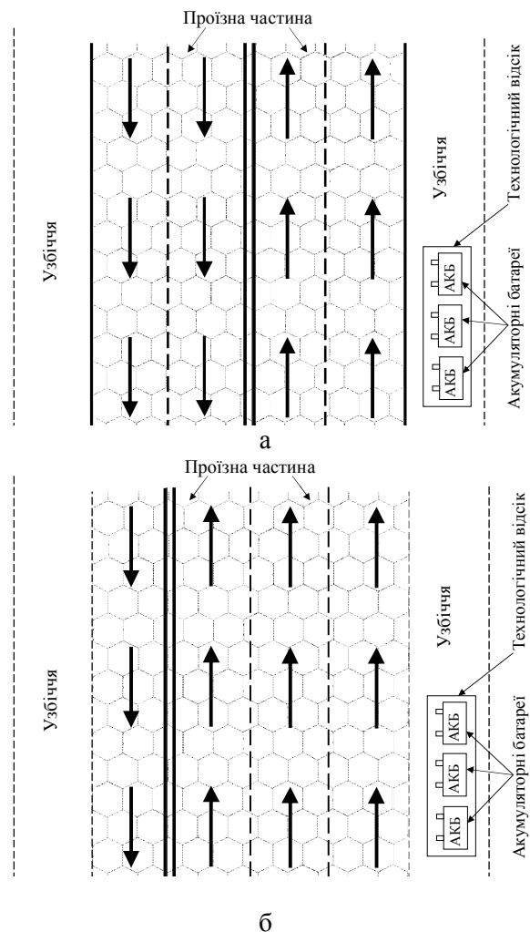
Рис. 3. Схема способу виконання дорожньої розмітки та автоматичного керування рухом автотранспортних засобів: а – дорожня розмітка при нормальних умовах; б – дорожня розмітка після регулювання для збільшення пропускної здатності у фронтальному напрямку
