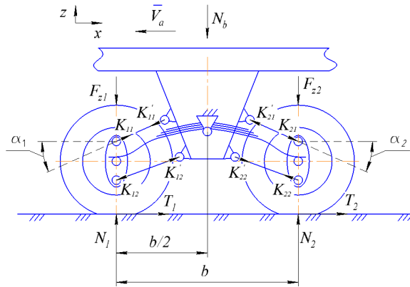
Рис. 2. Схема сил, которые действуют в балансирной тележке при торможении многоосного колесного транспортного средства: \vec{V}_a – вектор скорости движения КТС; N_1 и N_2 – нормальные реакции на соответствующих мостах балансирной тележки; T_1 и T_2 – соответствующие тормозные силы между шинами колес моста балансирной тележки и поверхностью дорожного покрытия; F_{z1} и F_{z2} – соответствующие усилия, передаваемые на мосты балансирной тележки через рессоры 2 (рис. 1); N_b – суммарное вертикальное усилие, действующее на балансирную тележку; \alpha_1 и \alpha_2 – соответственно углы наклона передних и задних направляющих рычагов балансирной тележки; K_{11} и K_{12} – реакции направляющих рычагов 3 (рис. 1) на передний мост тележки; K_{21} и K_{22} – реакции направляющих рычагов 4 на задний мост тележки; K'_{11} , K'_{12} , K'_{21} и K'_{22} – реакции, воздействующие на раму автомобиля со стороны направляющих рычагов
