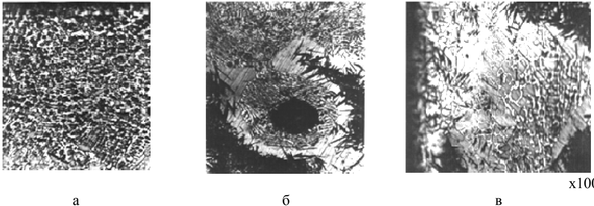
Рис. 1. Структурні складові зони оплавлення: а, б – ділянки білого чавуну; в – ділянка високовуглецевої сталі
