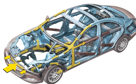
Рис. 5. Каркас автомобіля [17]
